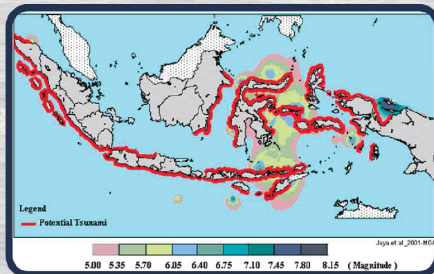
Peta Wilayah Potensial Bencana Tsunami di Indonesia
