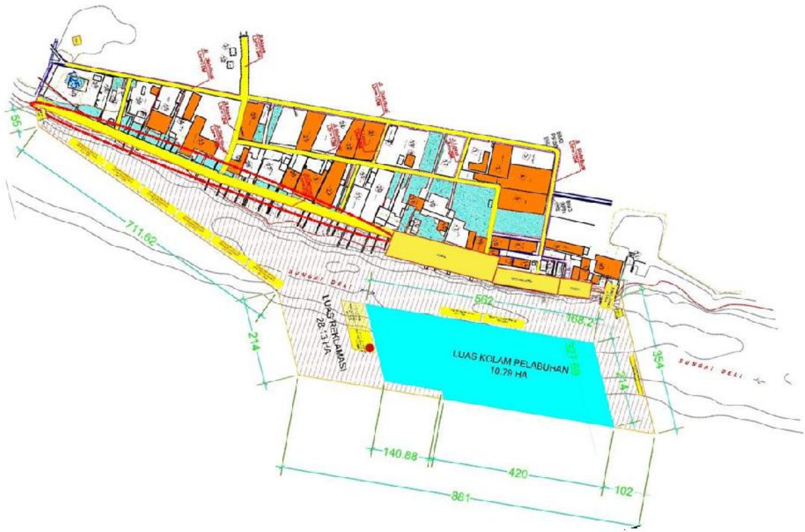
Gambar 45. Layout pengembangan PPS Belawan
