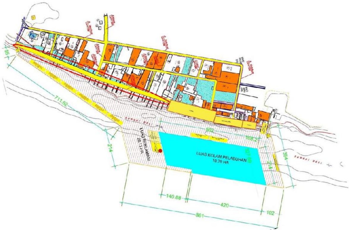
Gambar 44. Layout pengembangan PPS Belawan
