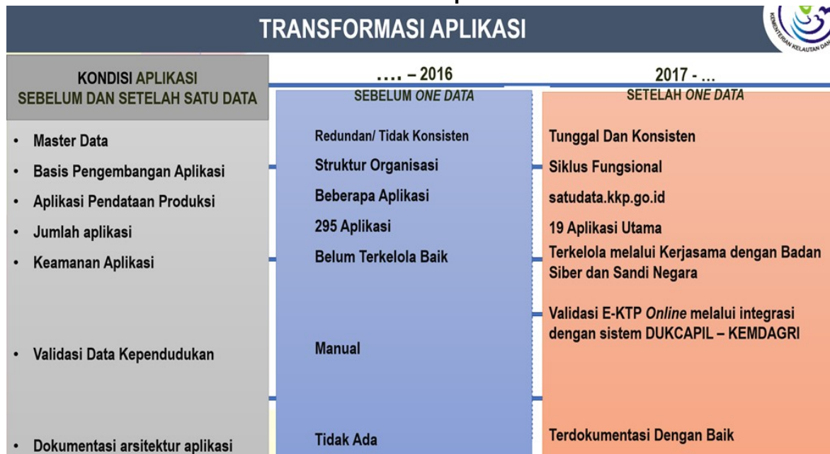
Gambar 4 Transformasi Aplikasi
