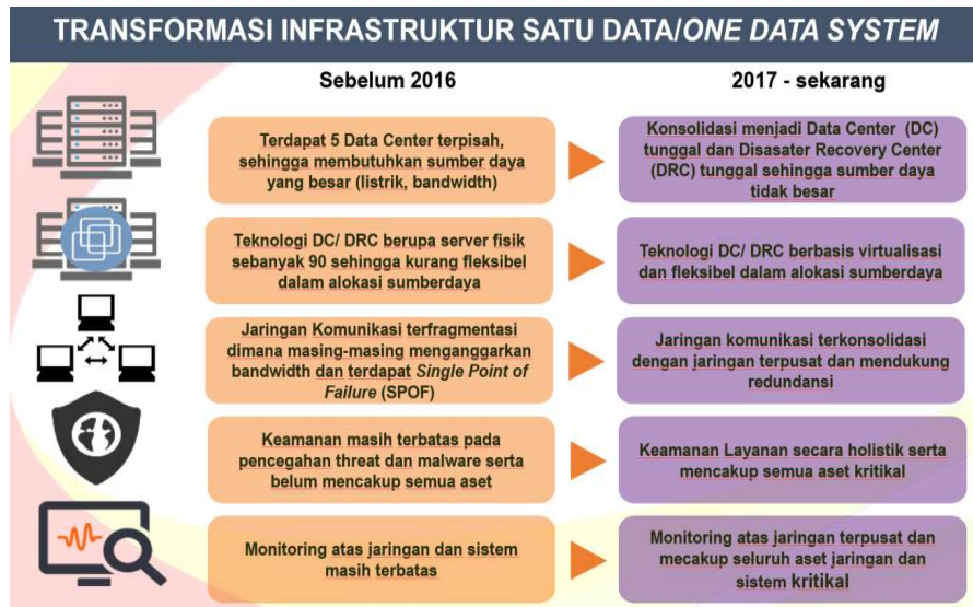
Gambar 4 Transformasi Aplikasi
