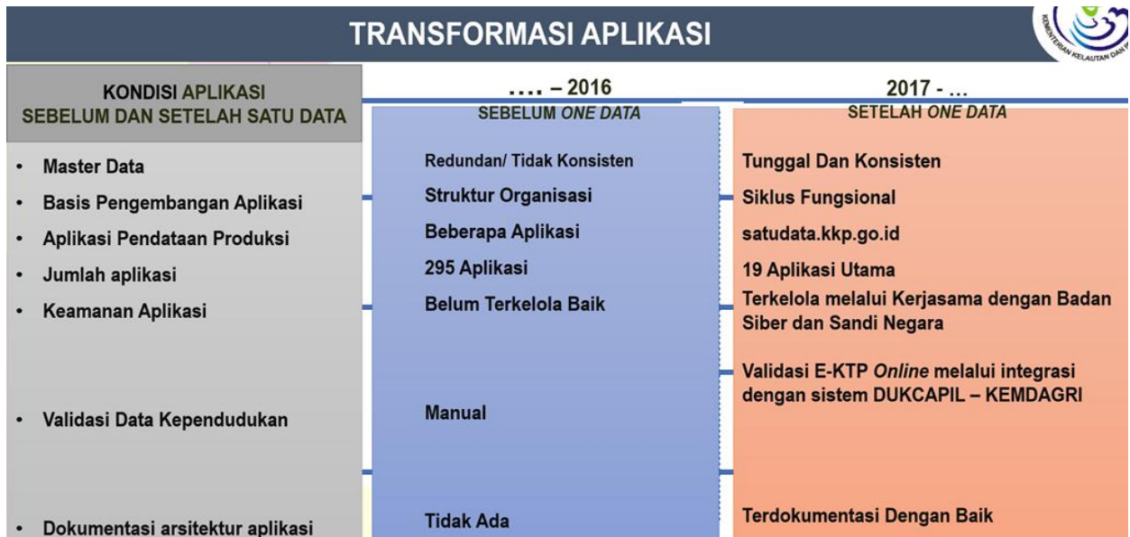
Gambar 4 Transformasi Aplikasi
