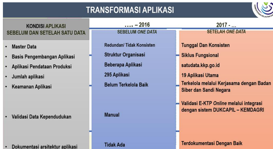
Gambar 3. Transformasi Aplikasi
