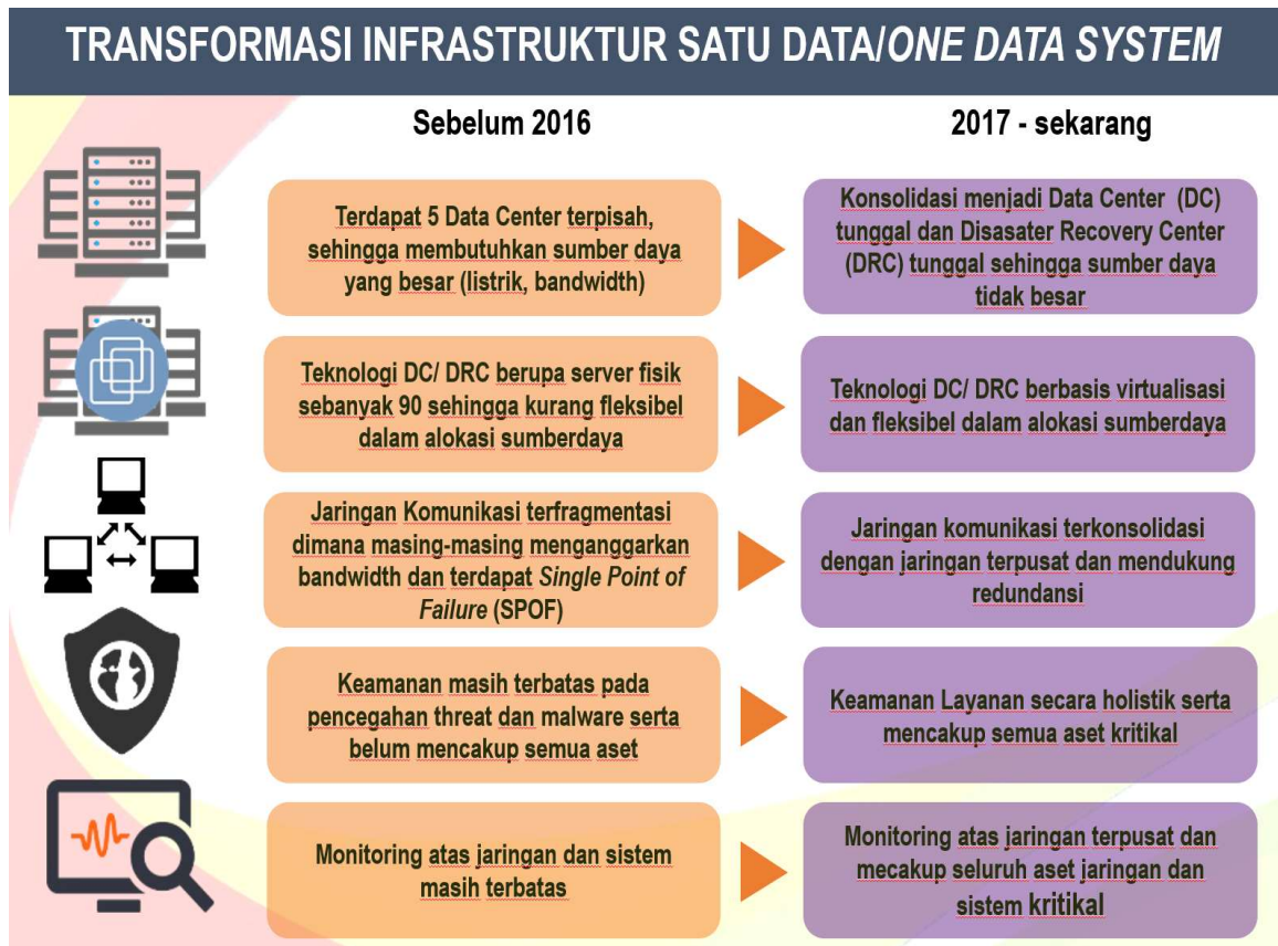
Gambar 4 Transformasi Aplikasi
