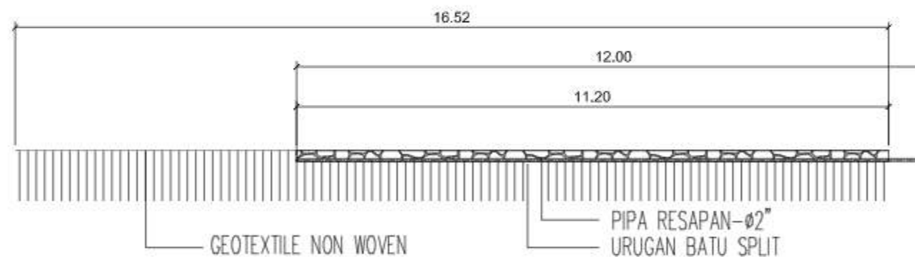
POTONGAN 2-2 SKALA 1 : 100
