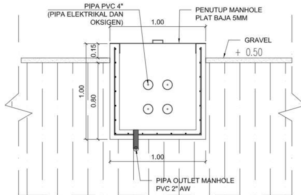
POTONGAN 1 - 1 SKALA 1 : 20
