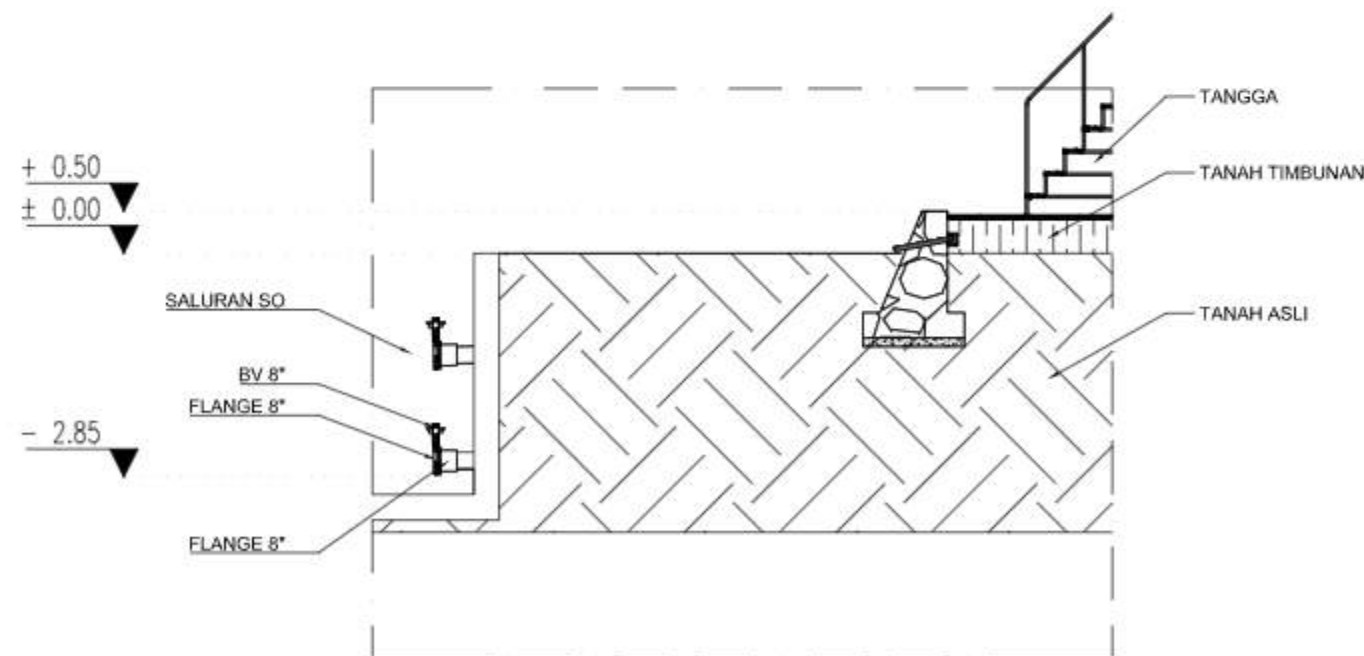
D.2 POTONGAN B - B
