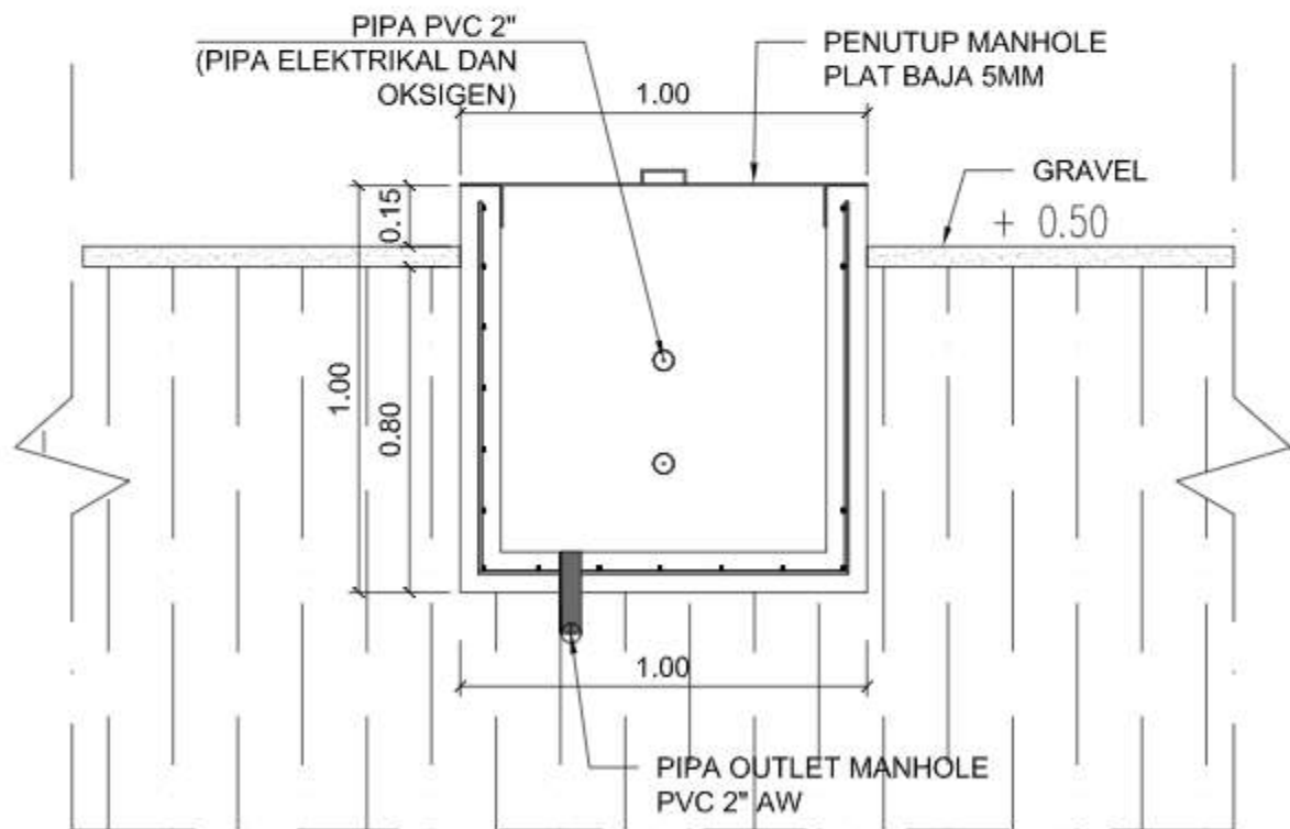
POTONGAN 1 - 1
