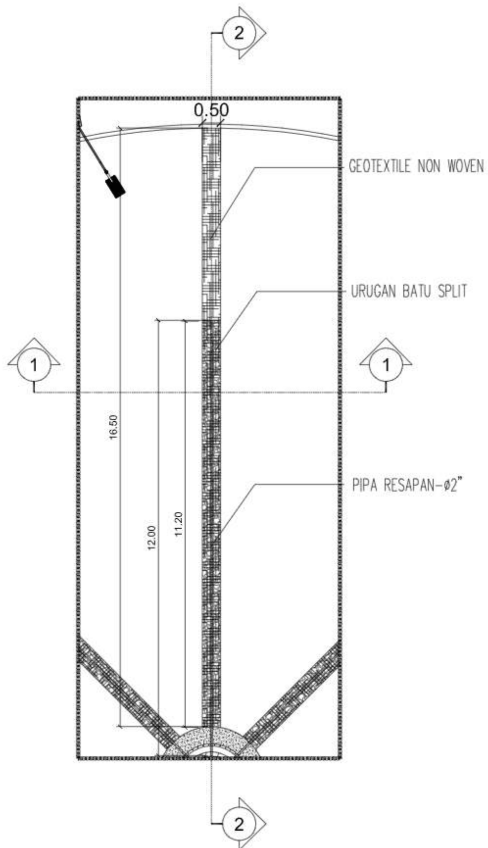
DETAIL - 03 SKALA 1 : 100
