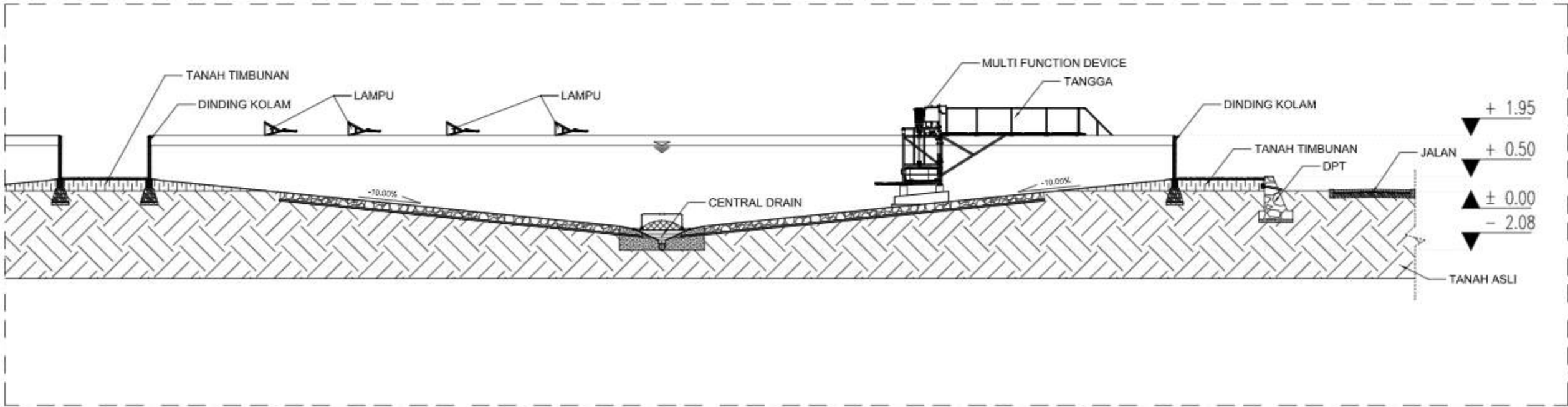
D.1 POTONGAN A - A SKALA 1 : 25
