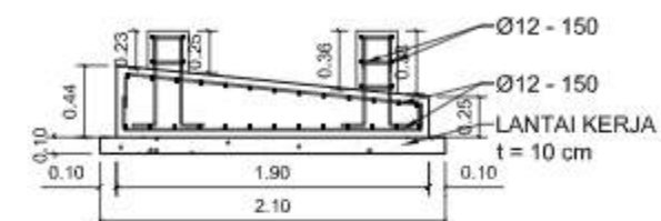
POTONGAN A - A
