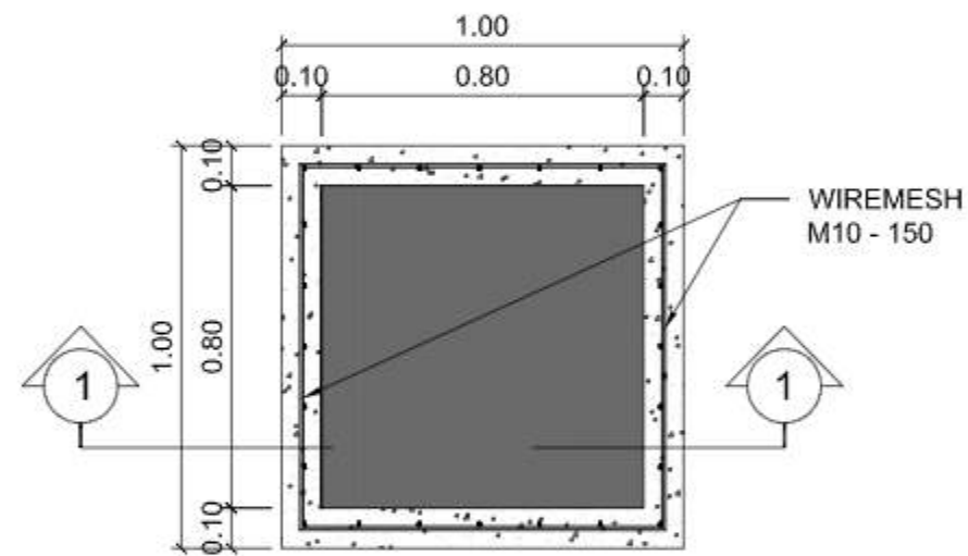
DENAH MANHOLE
