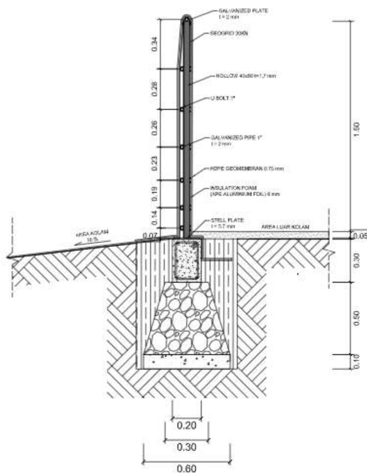
POTONGAN DINDING KOLAM SKALA 1 : 50
