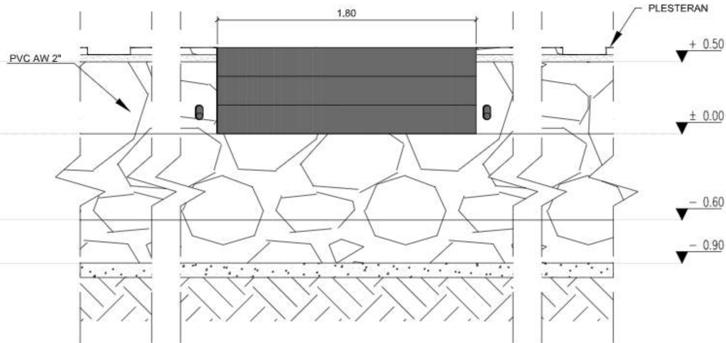
TAMPAK DEPAN TANGGA DPT
