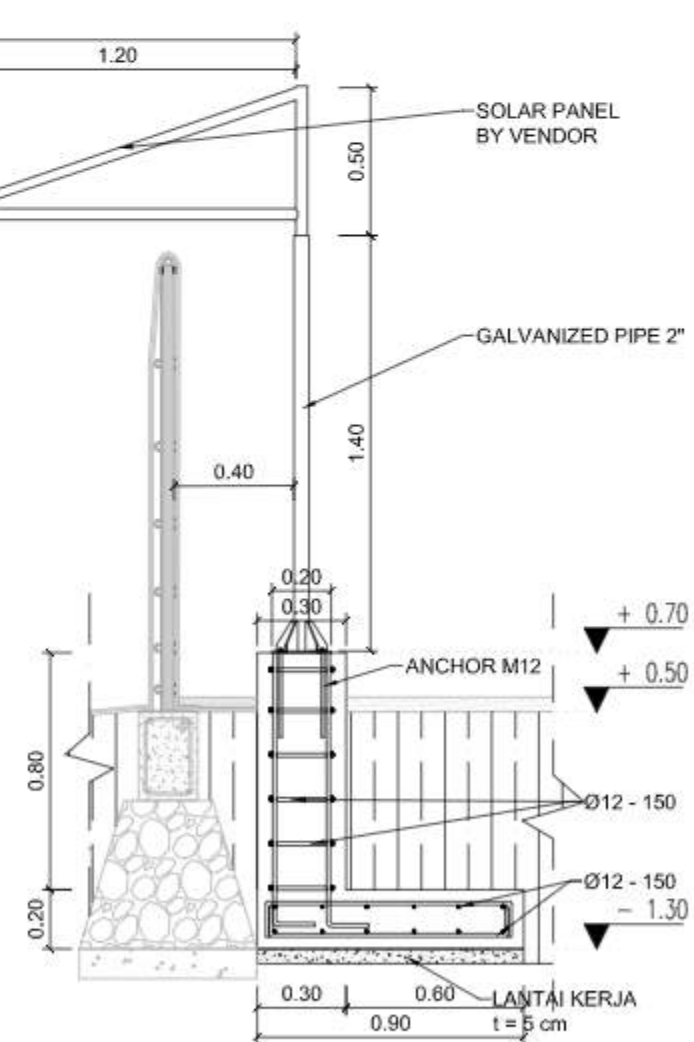
DETAIL POTONGAN PONDASI LAMPU
