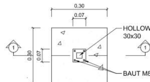
DENAH PONDASI TANGGA
