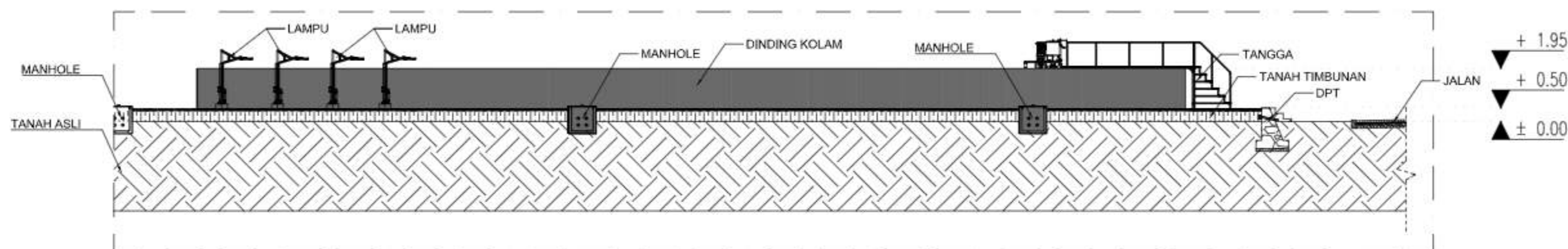
D.1 POTONGAN B - B
