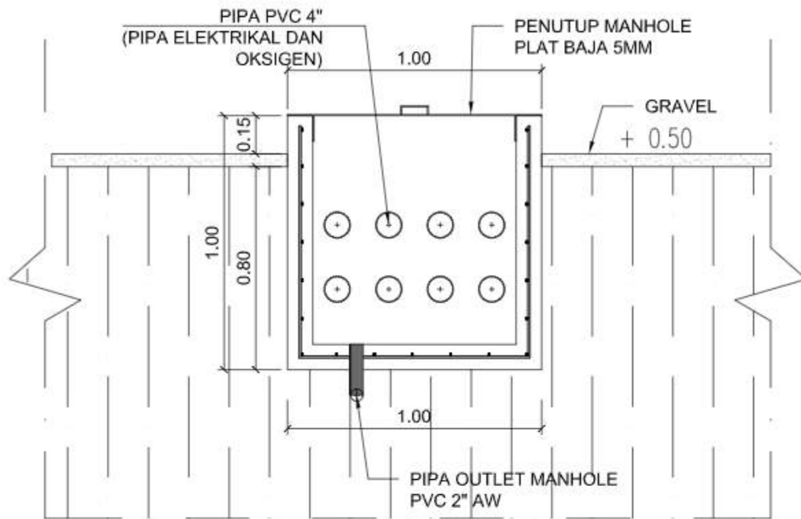
POTONGAN 1 - 1 SKALA 1 : 20
