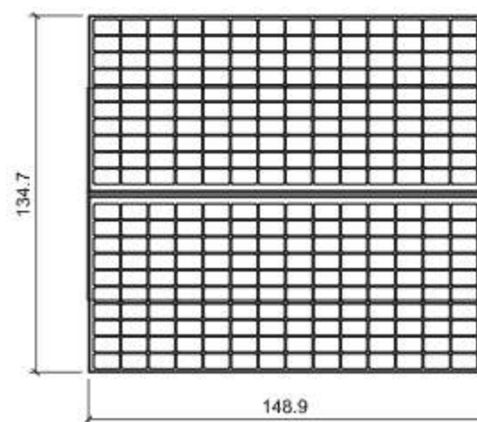
TAMPAK ATAS
