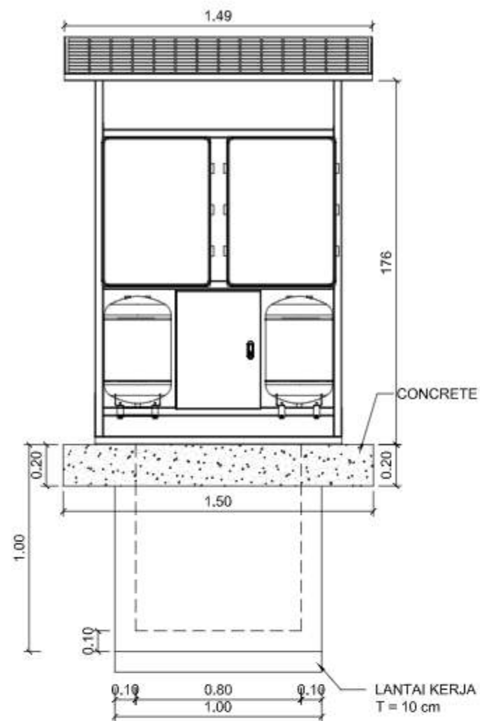
TAMPAK DEPAN
