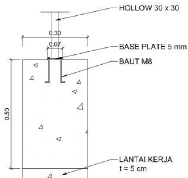
POTONGAN 1 - 1
