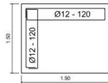
DETAIL PEMBESIAN
