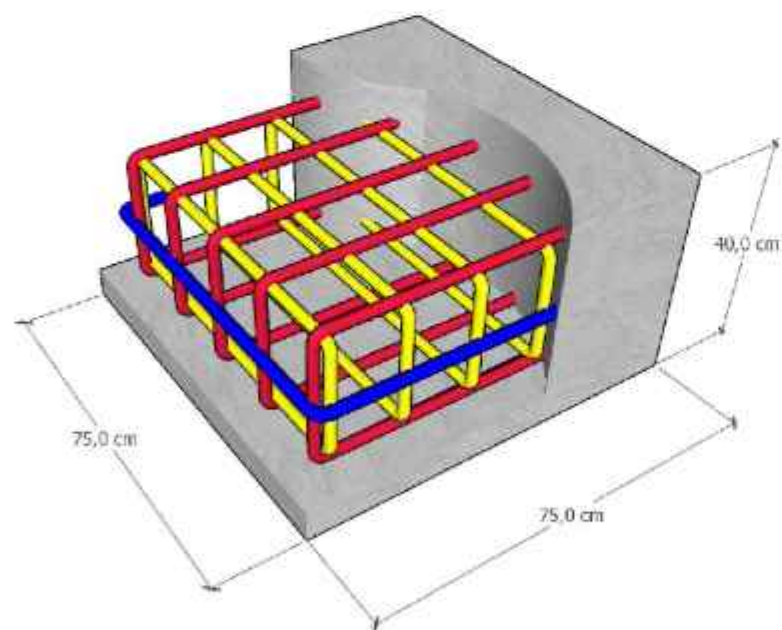
PERSPEKTIF POTONGAN BLOK BETON UK. 75X75X40 CM
