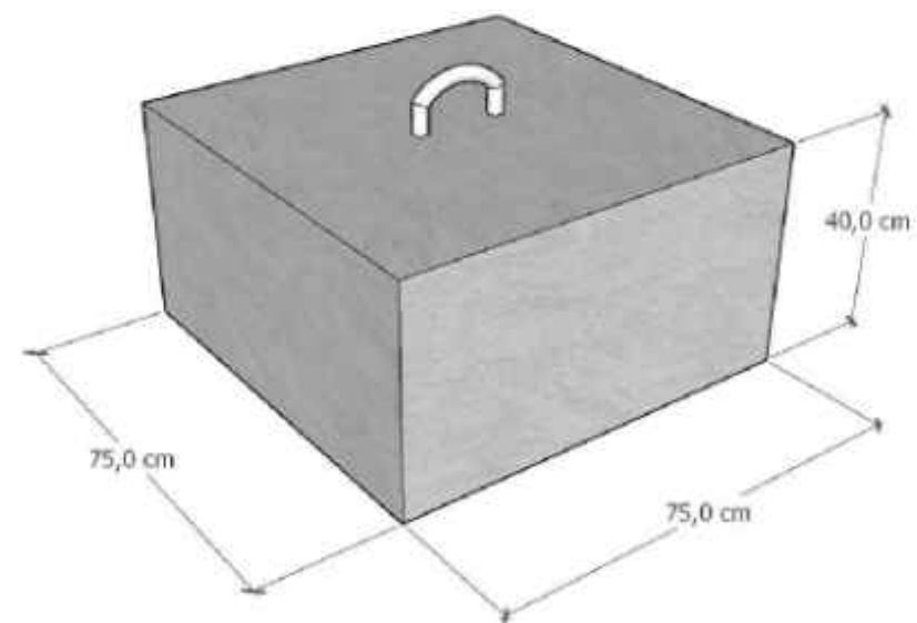
PERSPEKTIF BLOK BETON UK. 75X75X40 CM
