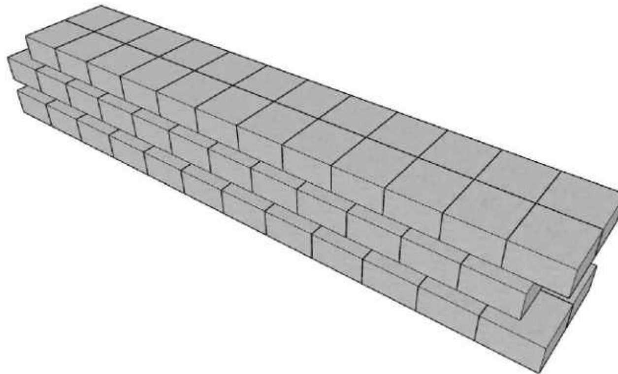
PERSPEKTIF MODUL PENYUSUNAN BLOK BETON UK. 75X75X40 CM
