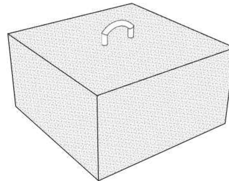
PERSPEKTIF BLOK BETON UK. 75X75X40 CM
