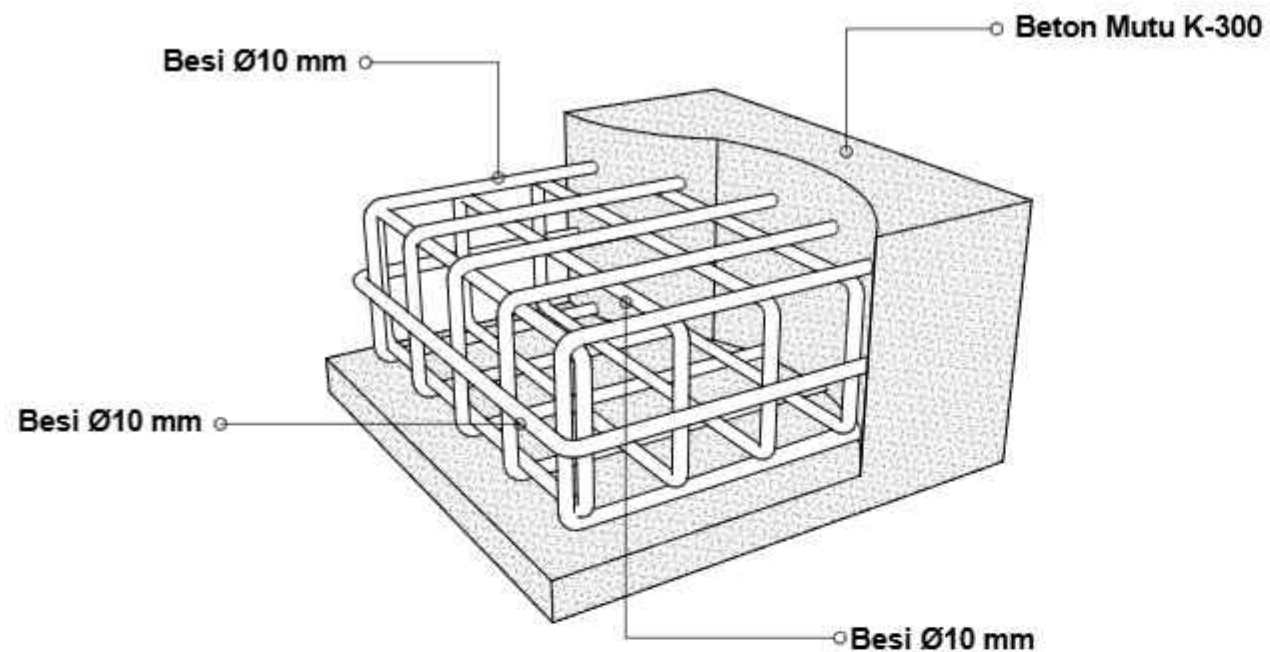
PERSPEKTIF POTONGAN BLOK BETON UK. 75X75X40 CM
