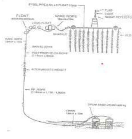
Gambar 10. Payoas Jepang (Kobayashi, 1988)
