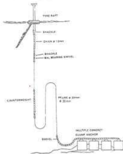
Gambar 18. Rumpon di Fiji
