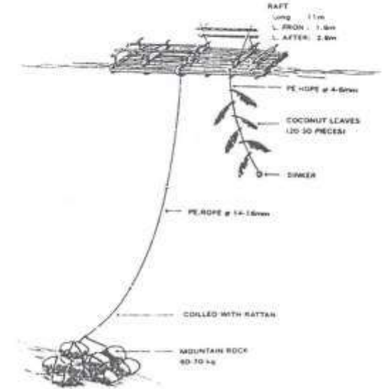
Gambar 23. Rumpon Mamuju Type Rakit Satu Susun (Dinas Perikanan Sulawesi Selatan, 1987)
