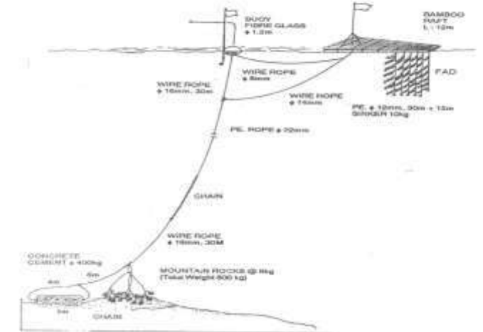
Gambar 7. Rompok Cakalang Milik PN. Perikani Aer Tembaga Bitung - Sulawesi Utara
