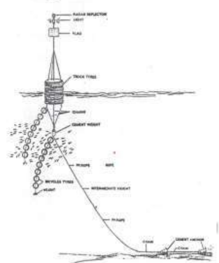
Gambar 21. Payoas yang Kembangkan Di Sri Lanka (Weerasoorya, 1987)
