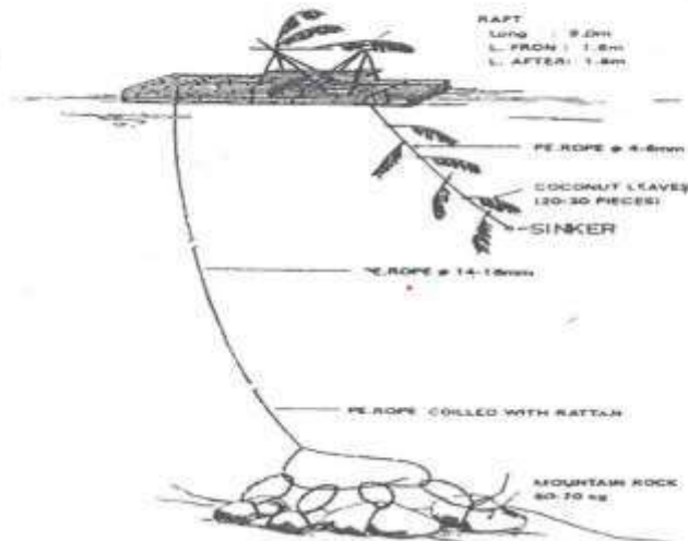
Gambar 24. Rumpon Mamuju Type Rakit Tiga Susun (Dinas Perikanan Sulawesi Selatan, 1987)
