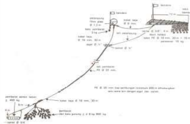
Gambar 5. Payaos Proyek Pembangunan dan Pengembangan Perikanan Sumatra Dengan Pelampung Fiberglass
