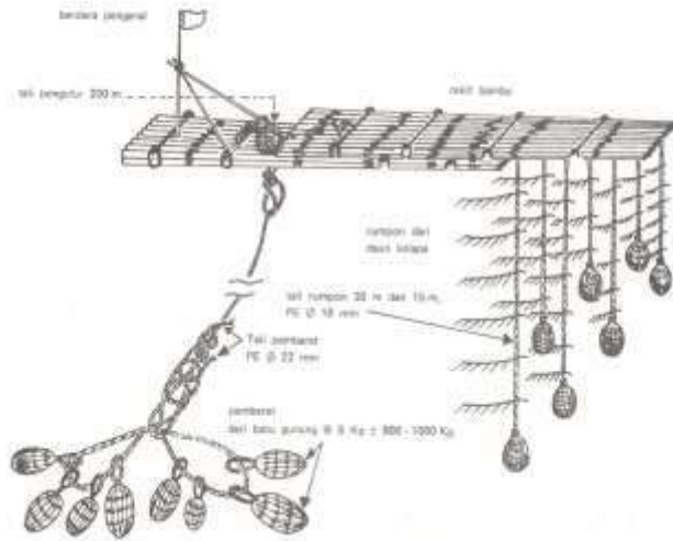
Gambar 2. Payaos Proyek Pembangunan dan Pengembangan Perikanan Sumatra
