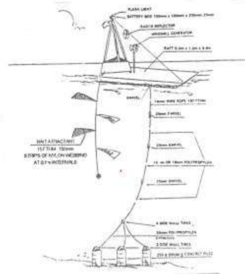
Gambar 17. Payoas yang dikembangkan di Pantai Barat Amerika
