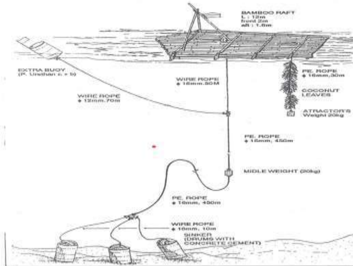
Gambar 6. Payaos Tipe KIHARA untuk Percobaan Di Laut Flores tahun 1981 (BPPI, Semarang)
